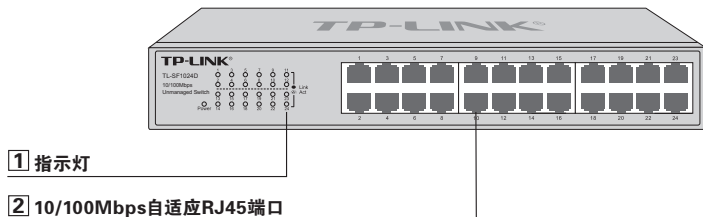
图1-1 前面板示意图
