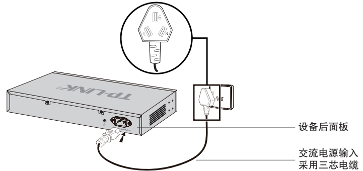
图2-5 PE线连接示意图
