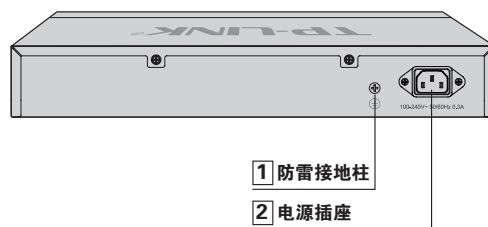
图1-2 后面板示意图
