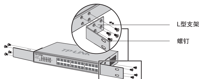
图2-2 L型支架安装示意图
